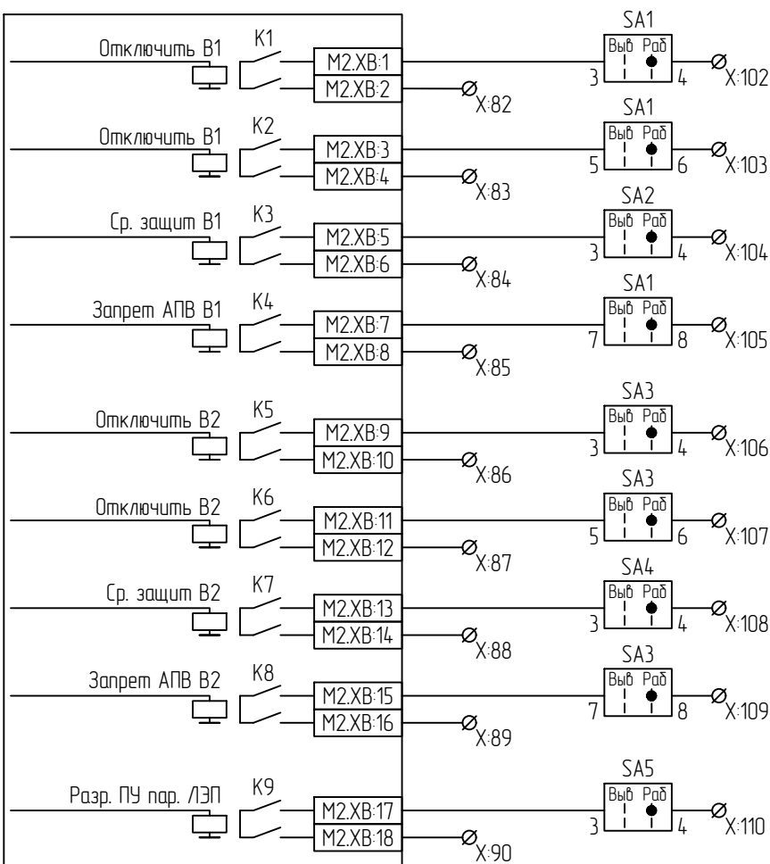
Выходные цепи
