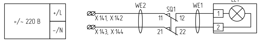
Цепи освещения шкафа
